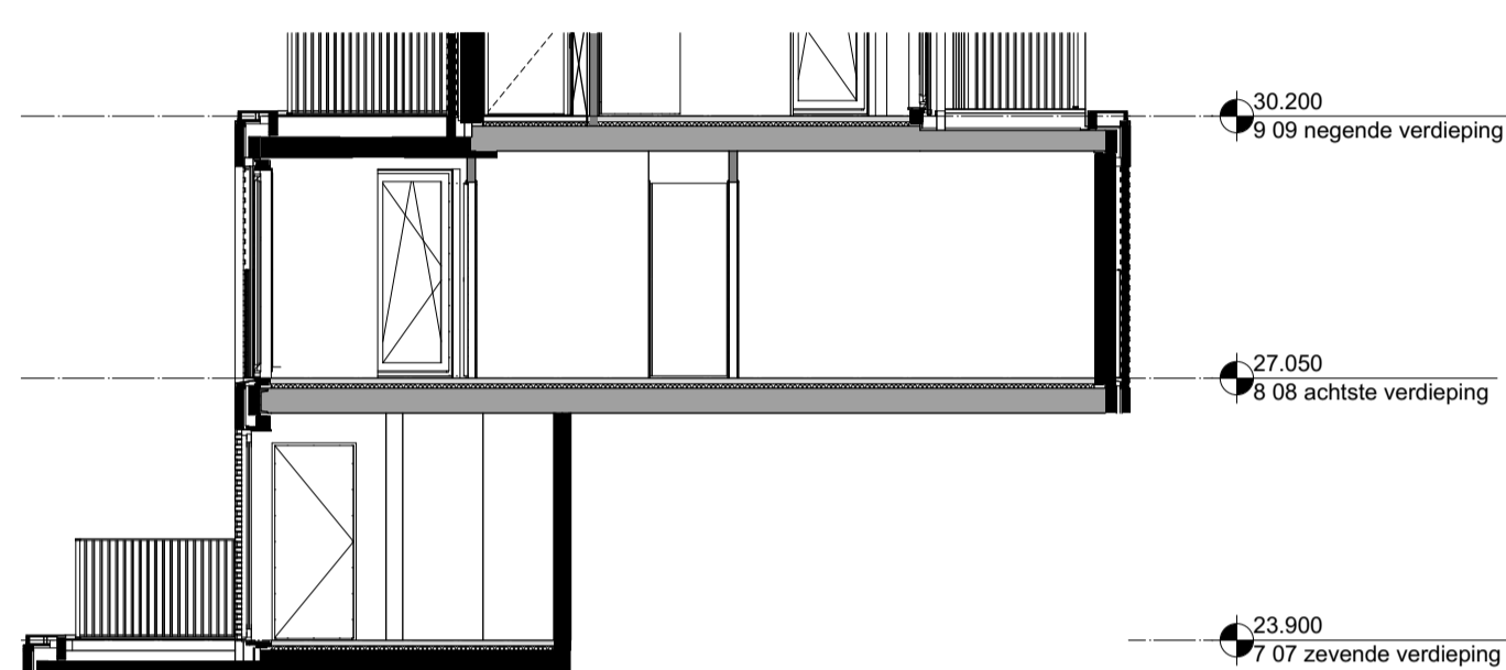
Doorsnede 1:100
