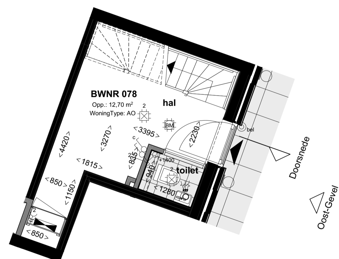
7e verdieping 1:50
