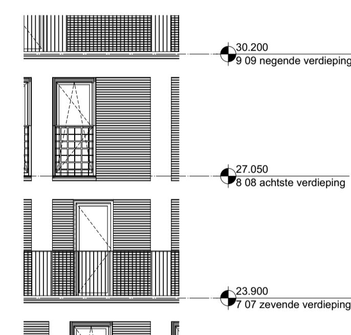
Oost-Gevel 1:100
