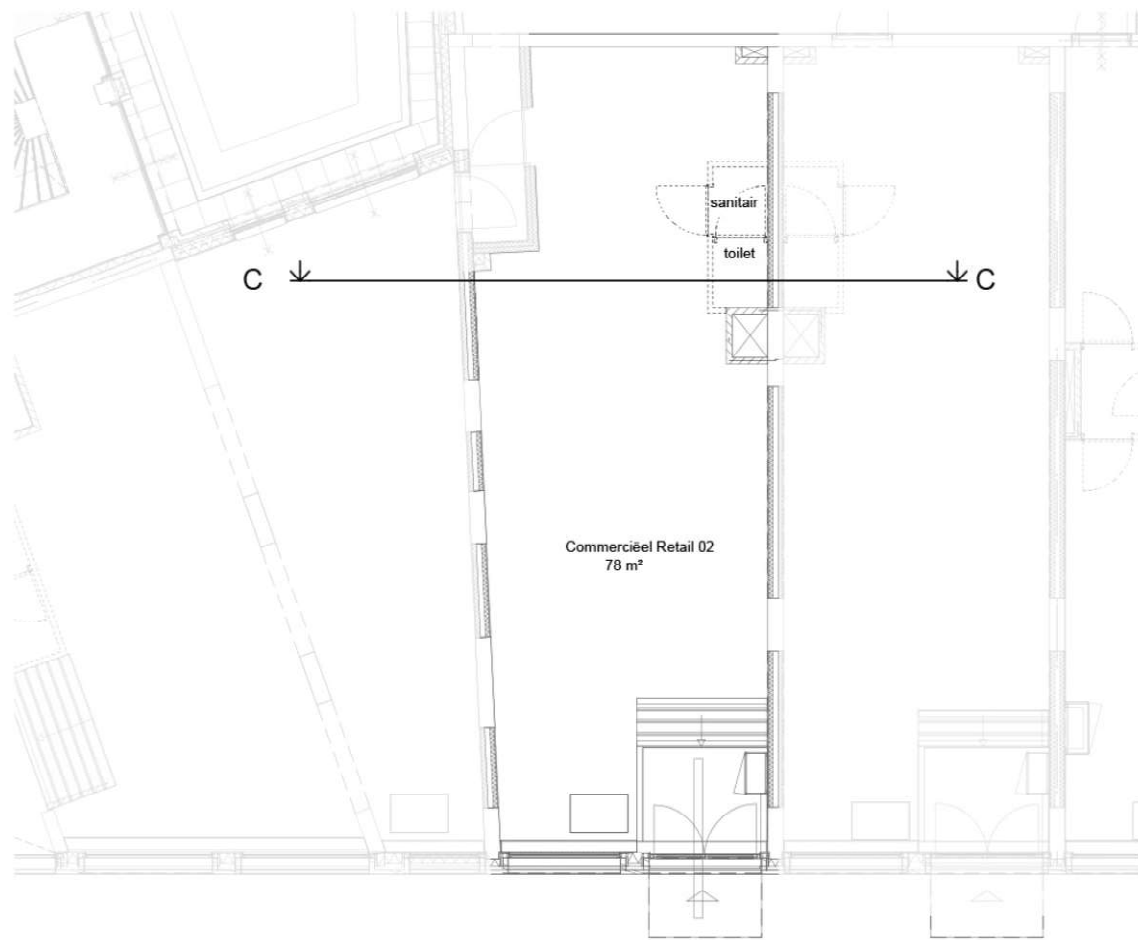
BEGANE GROND
