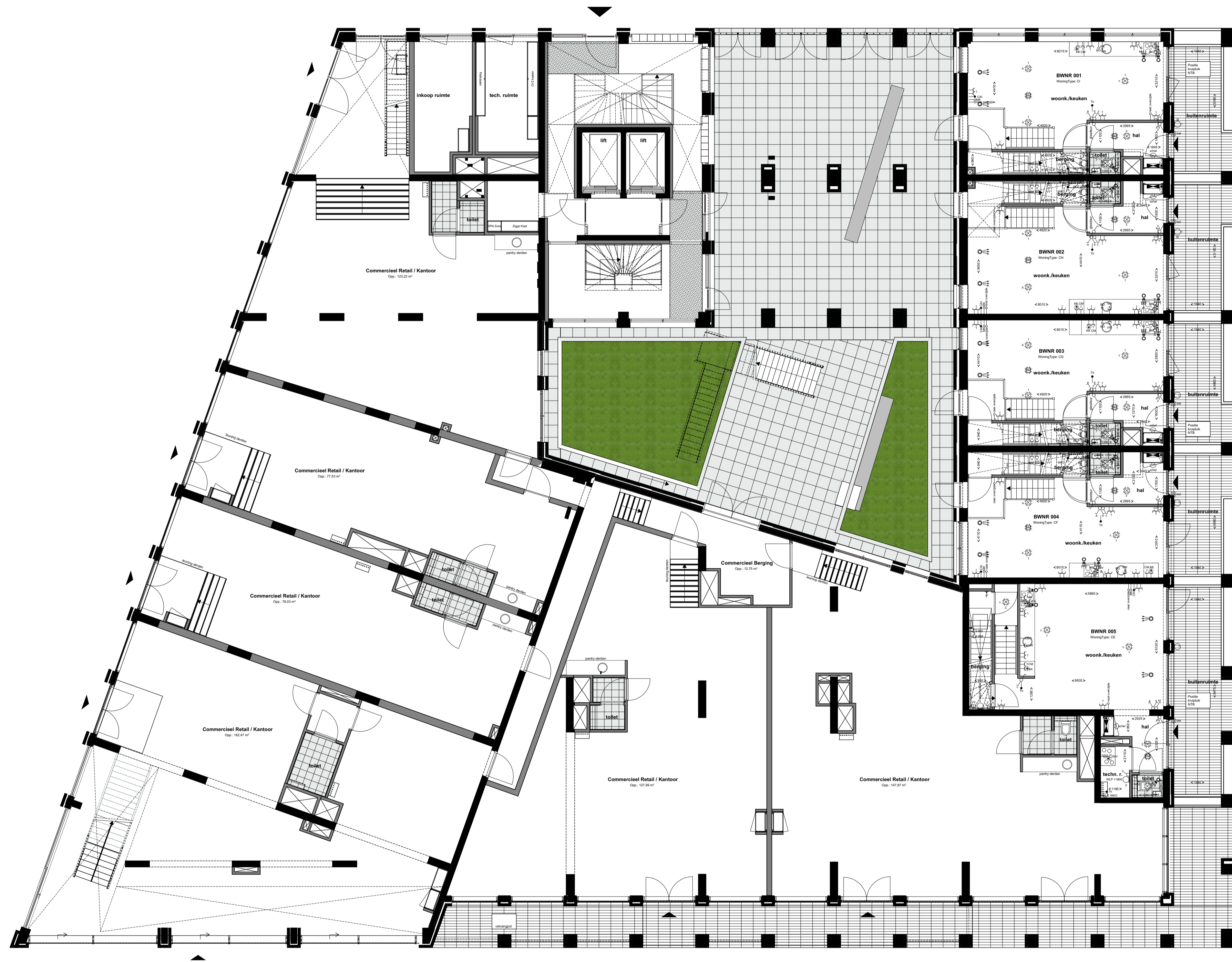
begane grond 1:100
