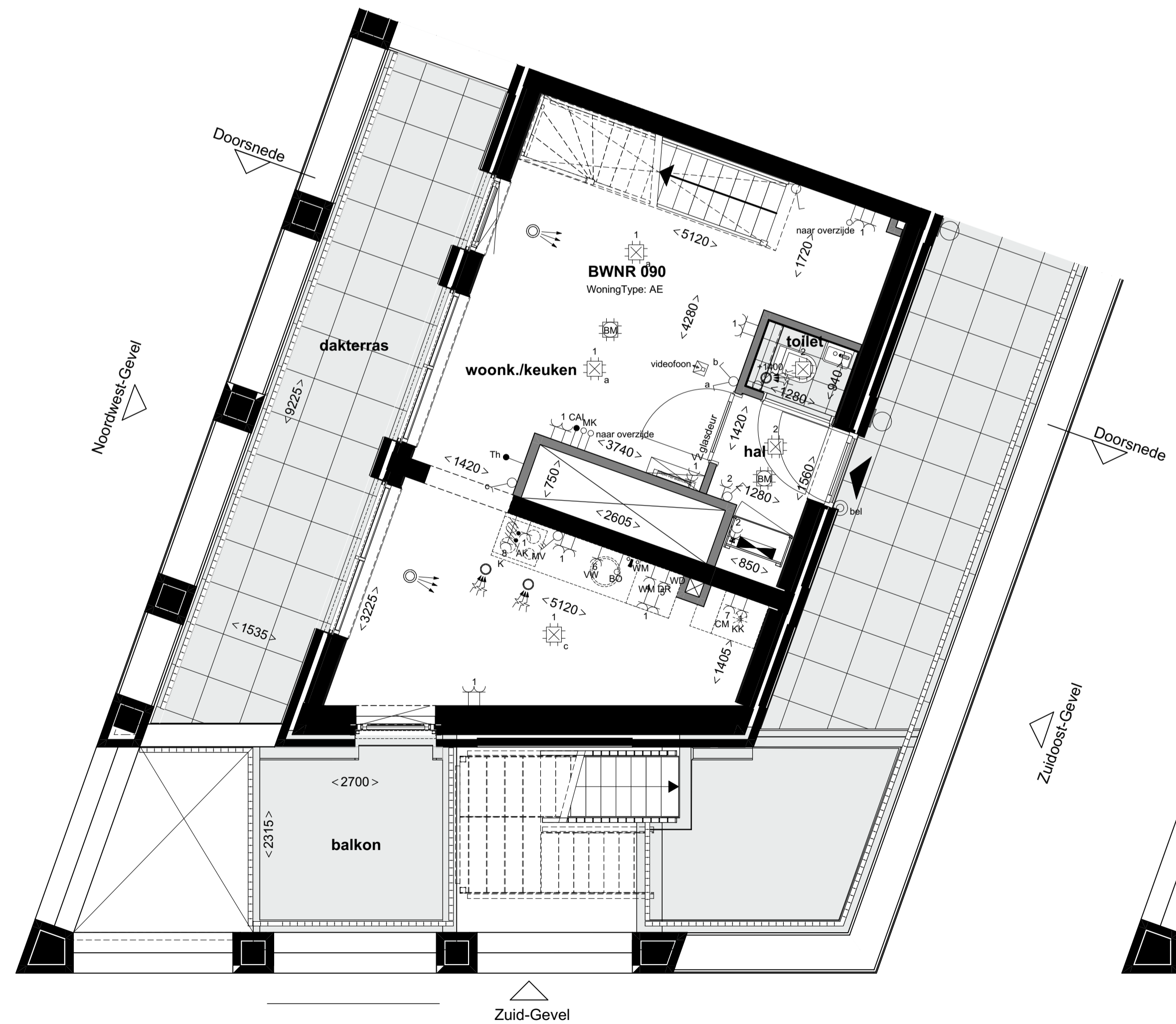
9e verdieping 1:50
