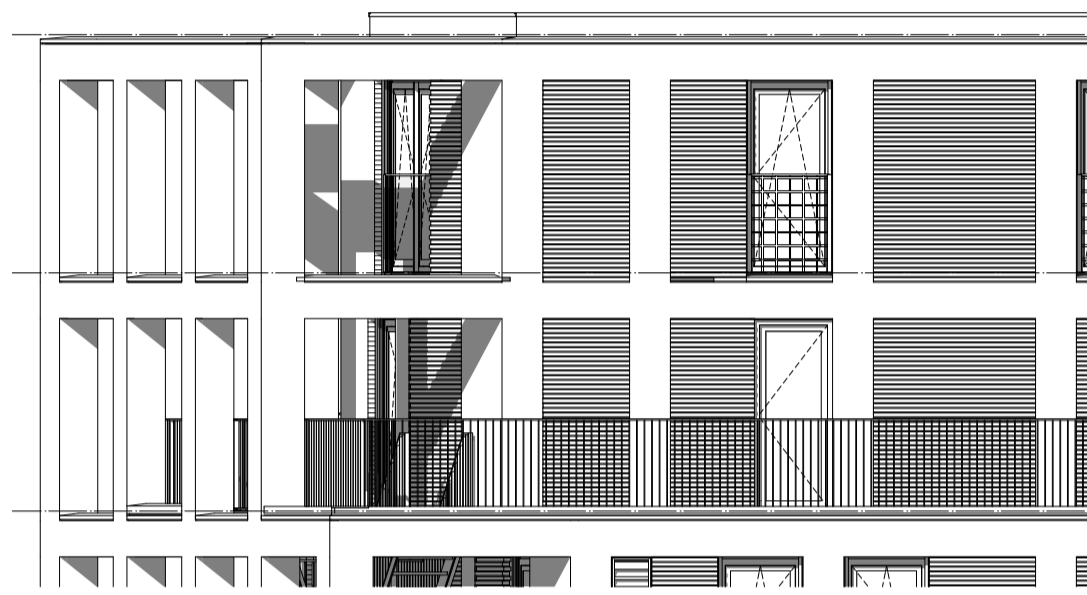
Oost-Gevel 1:100
