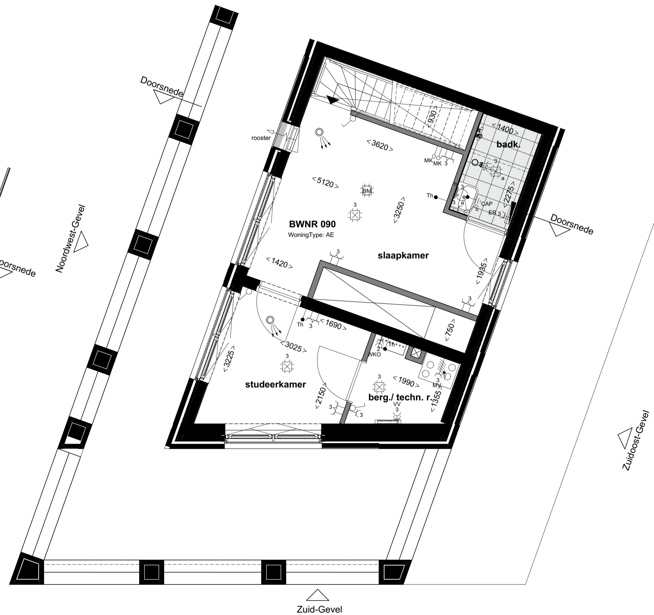
10e verdieping 1:50
