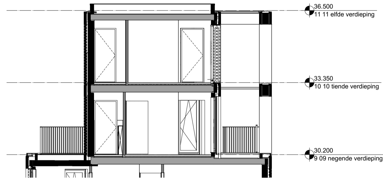
Doorsnede 1:100
